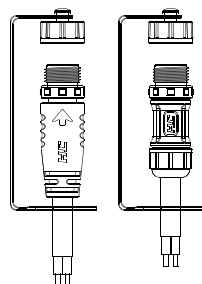
Schematic diagram of usage 安装示意图
