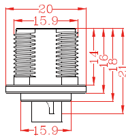
Regular style 常规款式 Mark: 01
