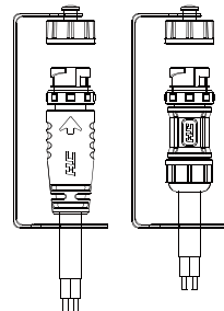
Schematic diagram of usage 安装示意图
