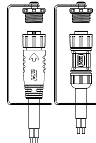
Schematic diagram of usage 安装示意图
