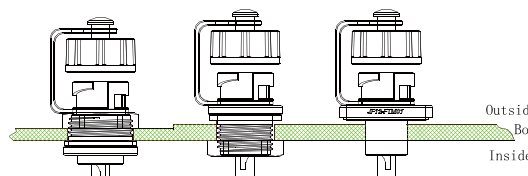
Schematic diagram of usage 安装示意图
