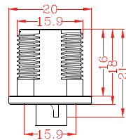
Extended style 加长款式 Mark: 02
