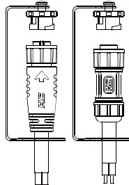
Schematic diagram of usage 安装示意图
