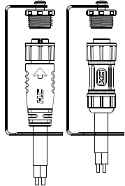
Schematic diagram of usage 安装示意图
