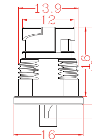
Extended style 加长款式 Mark: 02
