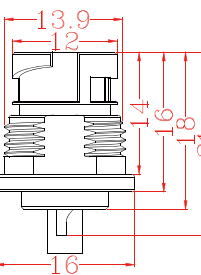
Regular style 常规款式 Mark: 01
