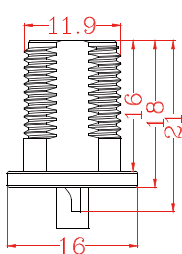
Extended style 加长款式 Mark: 02
