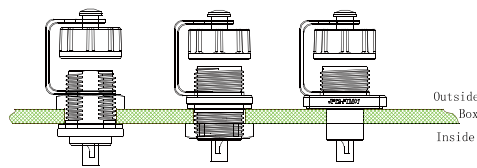
Schematic diagram of usage 安装示意图
