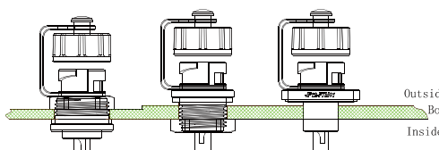
Schematic diagram of usage 安装示意图
